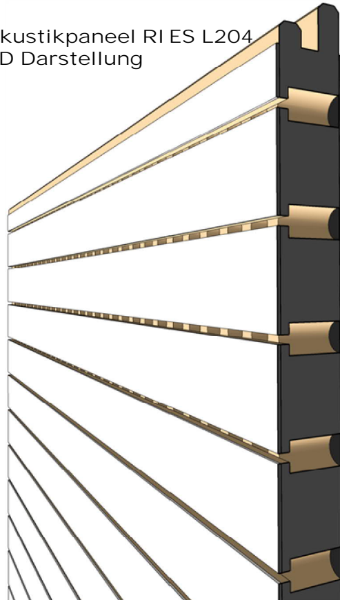
Akustikpaneel RI ES L204 Bemusterung: Trägerplatten Multiplex Furnier: Birke Oberfläche: Klar lackiert
